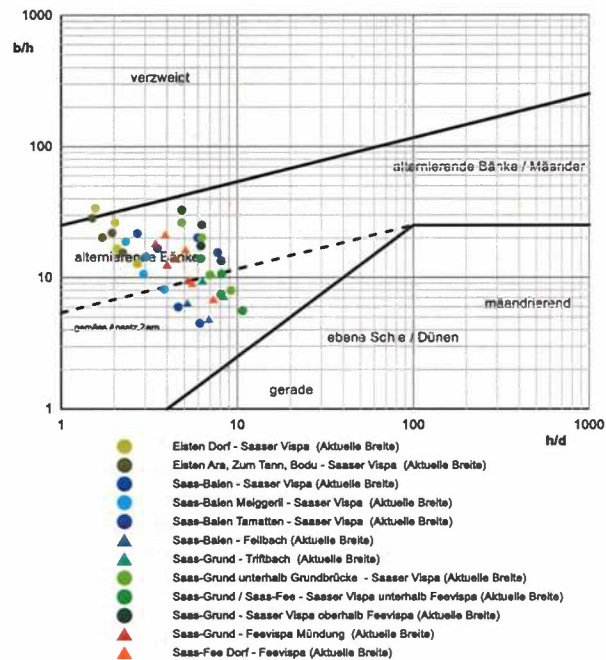
Abb. 2 Überblick über die heutigen morphologischen Verhältnisse (daSilva-Diagramm, h: Abflusstiefe, d: mittlerer Korndurchmesser und b: Sohlenbreite). Pro Gewässerabschnitt sind zwischen 2-4 Datenpunkte eingetragen, um der Bandbreite des relevanten Abflusses (HQ2, resp. HQ5) und der variierenden Breite im IST-Zustand Rechnung zu tragen.
