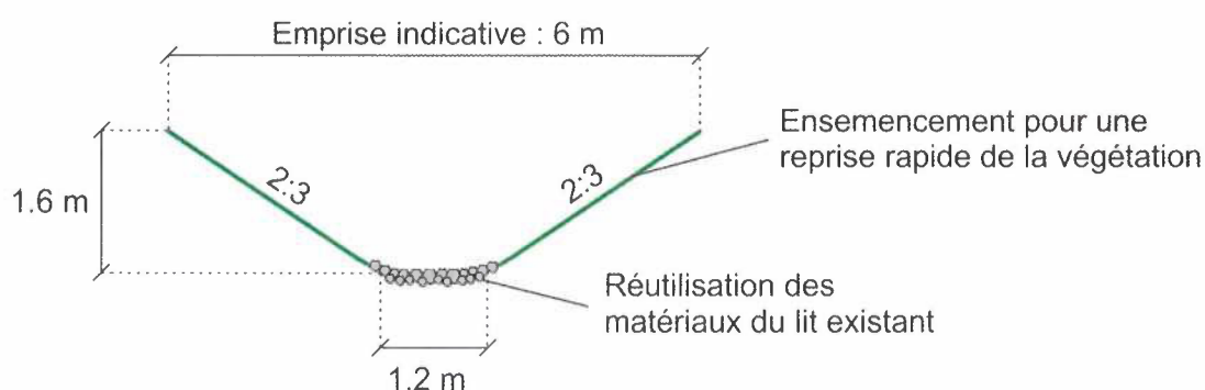
Figure 7 : Section (coupe schématique) à aménager pour garantir le transit des blocs et coulées de boue (cf. situation en figure 6).
