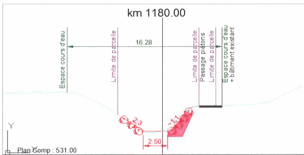
Figure 12 : Profil type d'aménagement de la Rèche au niveau de l'Impasse de la Cascade
