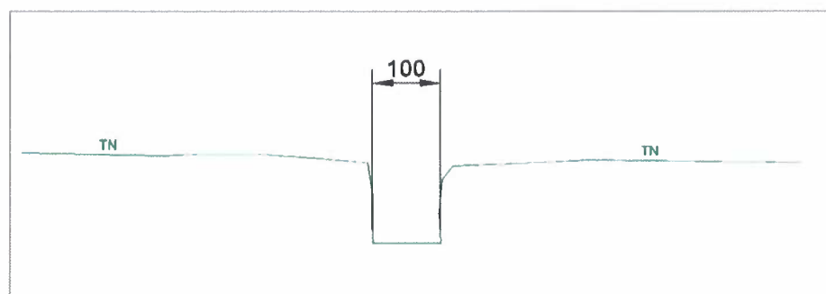
Figure 5 : Profil en travers du torrent du Taillis, tronçon naturel, en amont de la rue des Harroz
