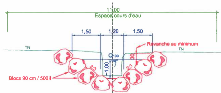
Figure 24 : Profil type d'aménagement du torrent du Taillis
