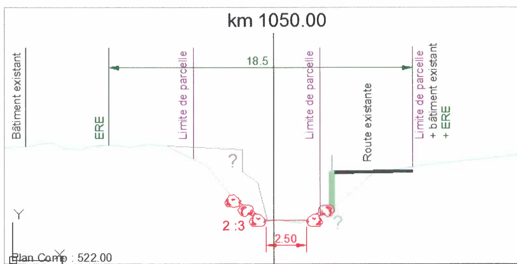
Figure 11 : Profil type d'aménagement de la Rèche en aval de la passerelle
