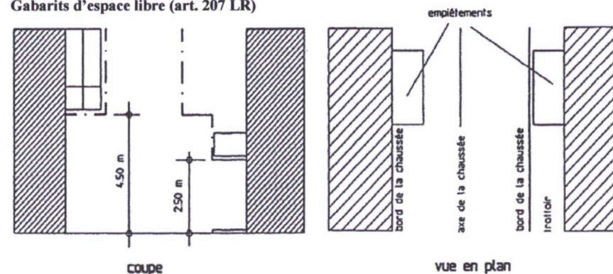
Gabarits d'espace libre (art. 207 LR)
