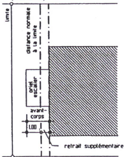
Empiètement de plus de 1,00 m. (art. 22 LC)
