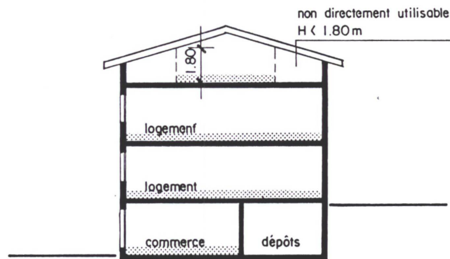
coupe
