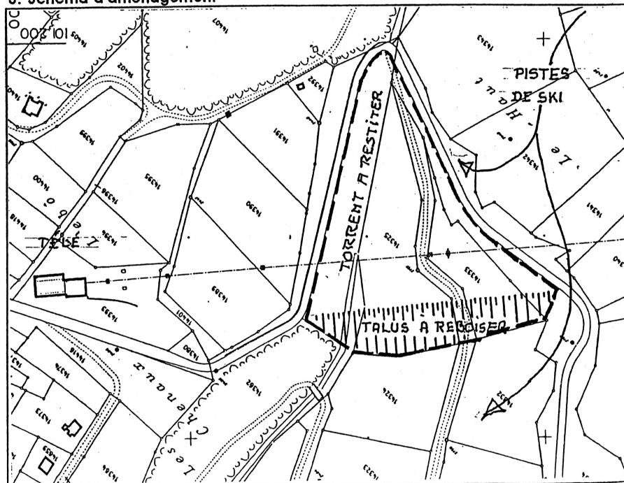
3. Schéma d'aménagement
